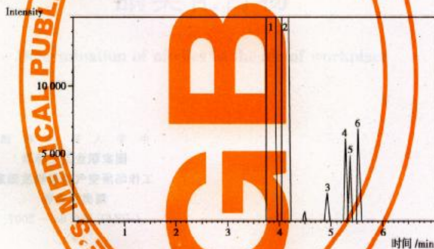
图 1 标准色谱图
